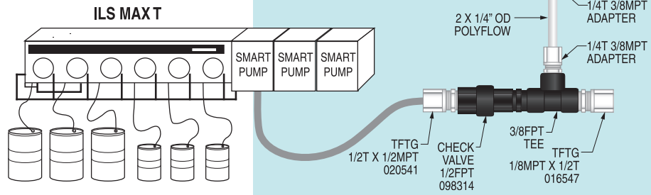
ILS Max Air Valve Plumbing
